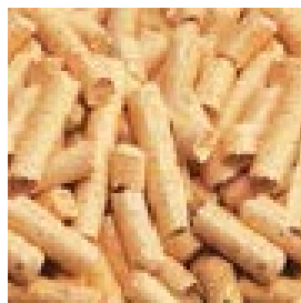
Пеллеты
