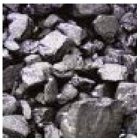
Каменный уголь
